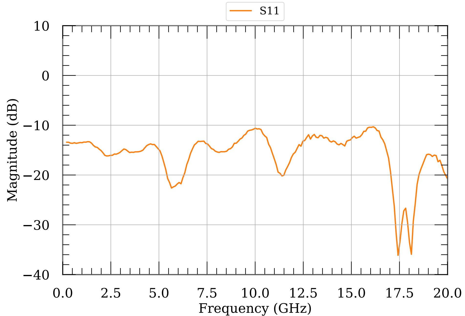
LNA S-params module079v2
